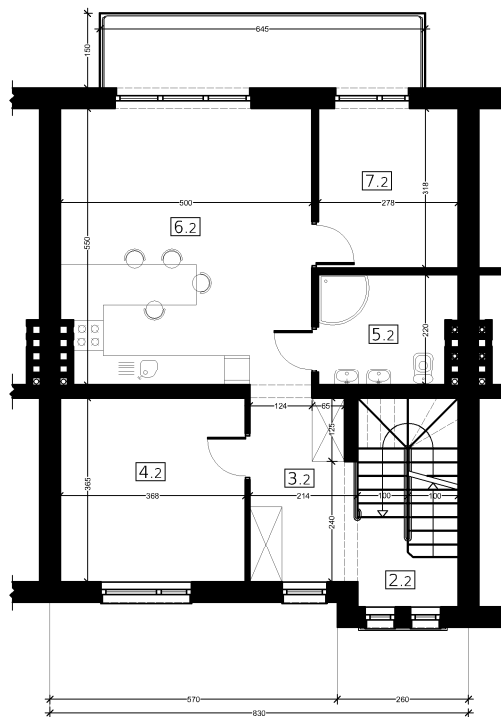
PIĘTRO
